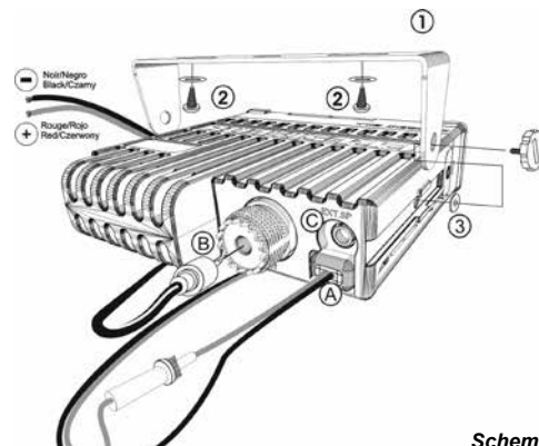
Schemat montażu
