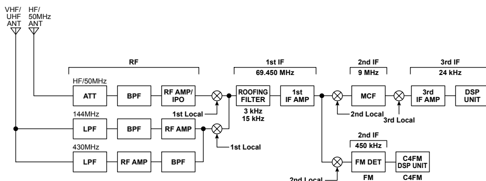
SCHÉMA FONCTIONNEL DES ÉTAGES D'ENTRÉE
