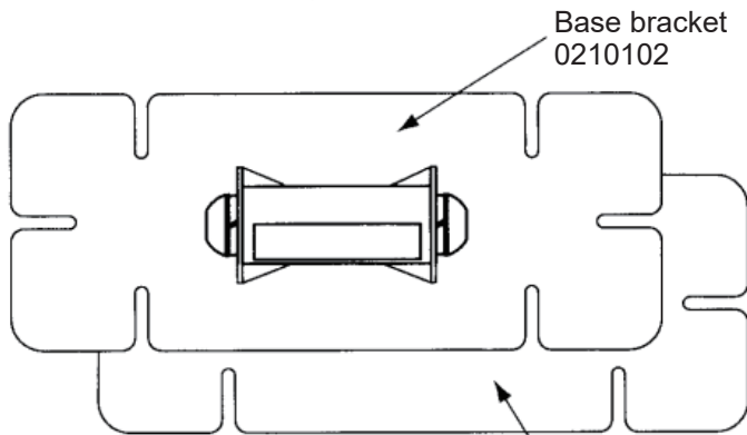
Spring 0210104
